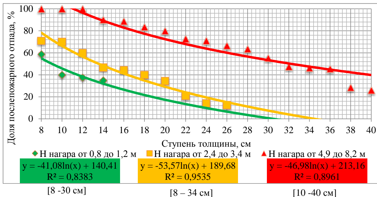
Рис. 3. Шкала доли потенциального отпада деревьев сосны по густоте в сосняках сухих типах леса ( C_2 ) пройденных низовыми пожарами с различной высотой нагара
